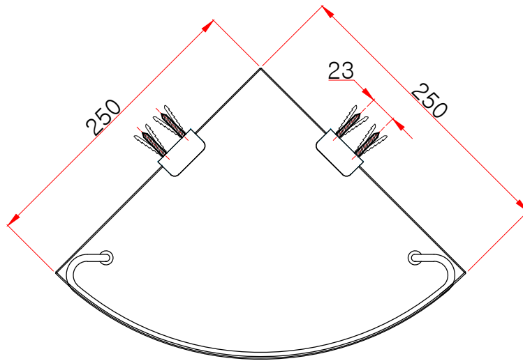
평(윗)면도
