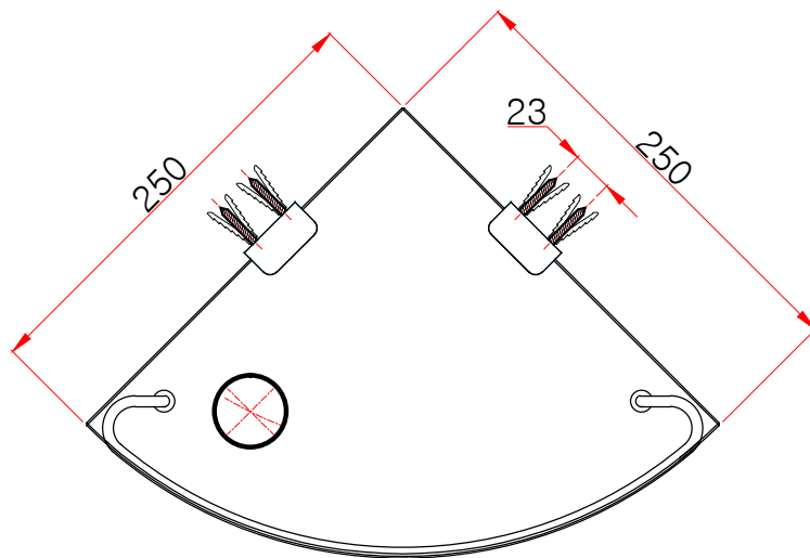
평(윗)면도
