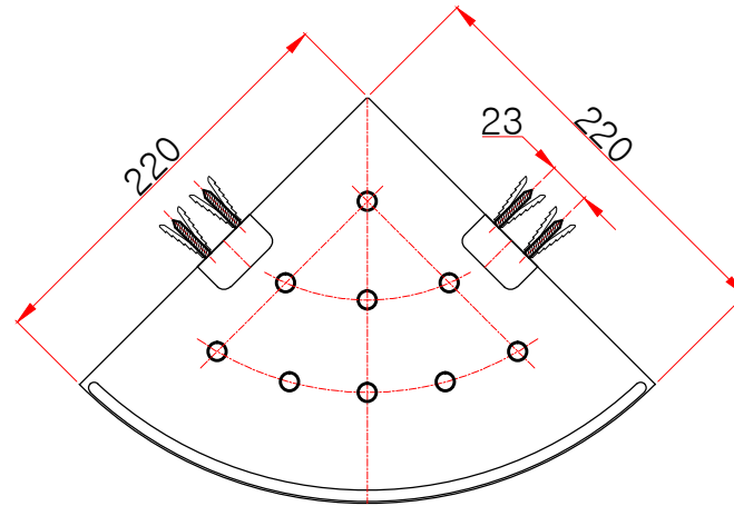
평(윗)면도
