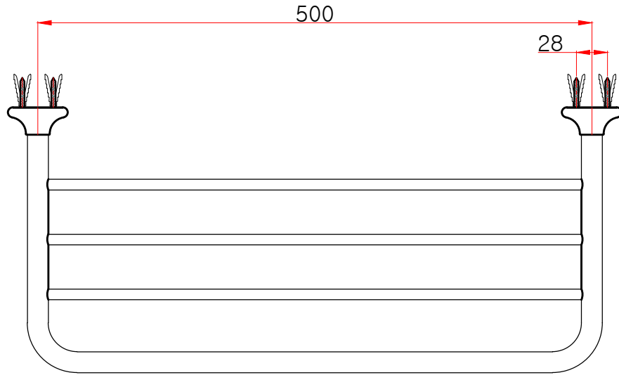
평(윗)면도
