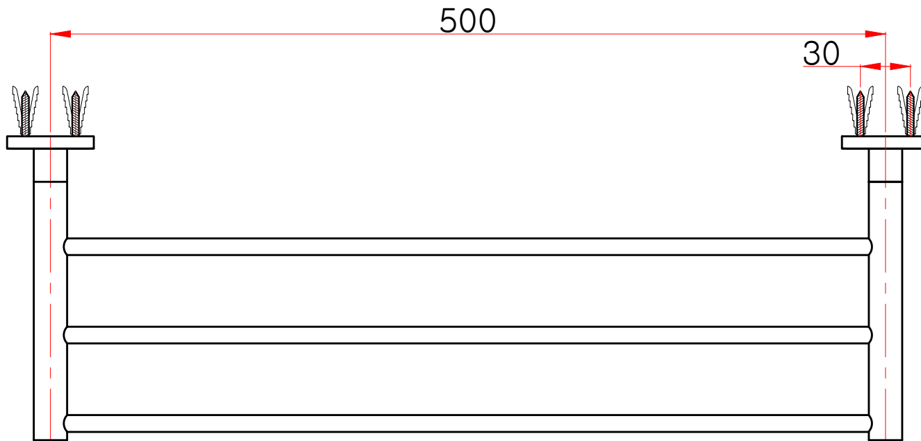
평(윗)면도
