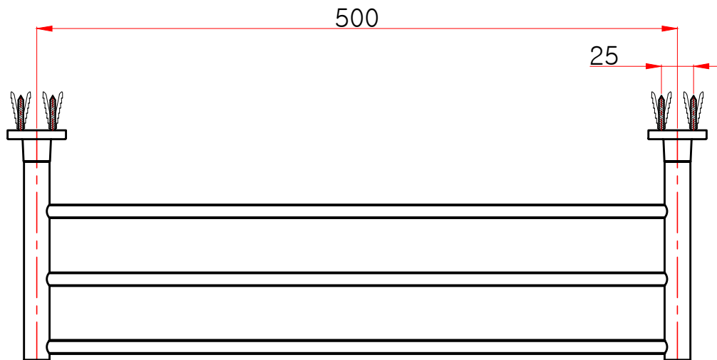
평(위)면도
