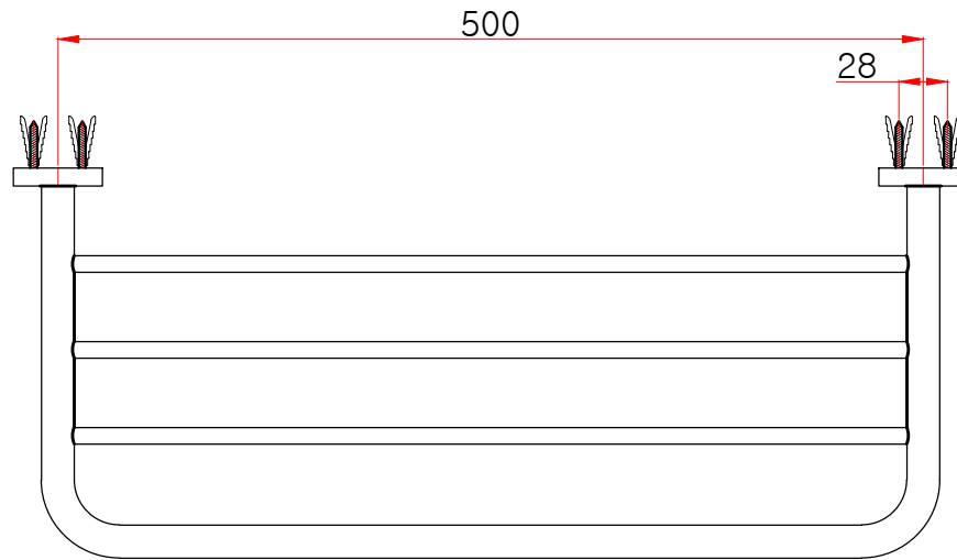
평(윗)면도
