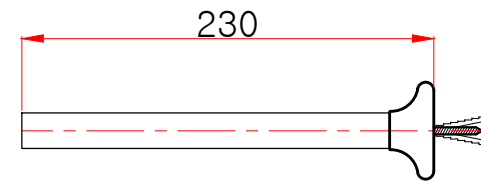
측면도
