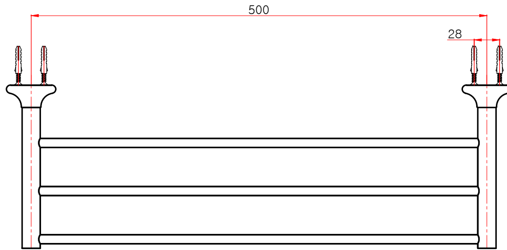
평(위)면도
