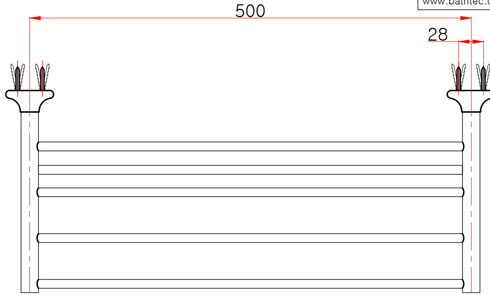
평(윗)면도
