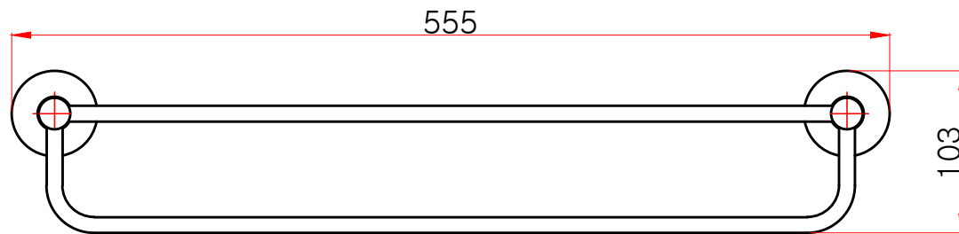
정면도
