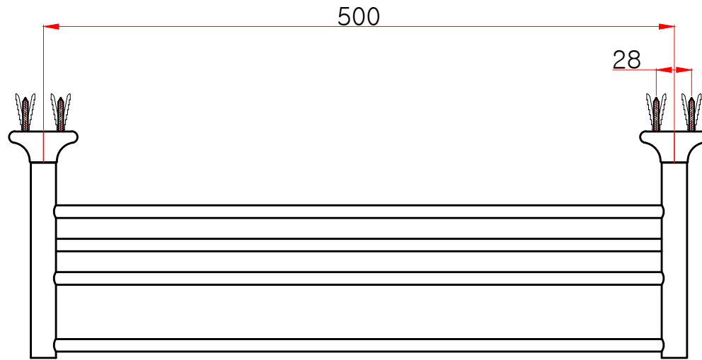
평(윗)면도
