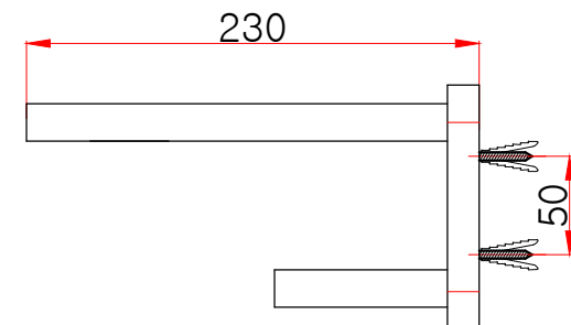
측면도
