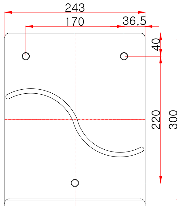
정면도
