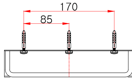
평(윗)면도
