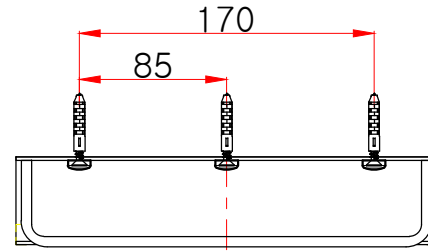
평(윗)면도
