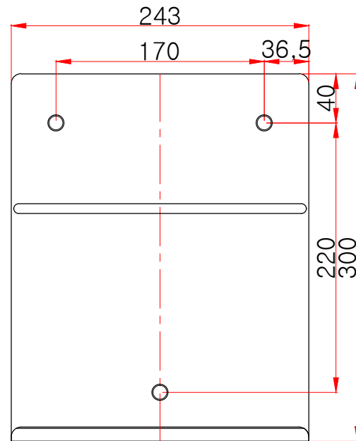
정면도
