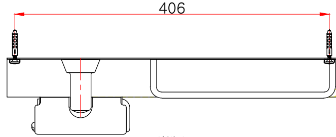
평(윗)면도
