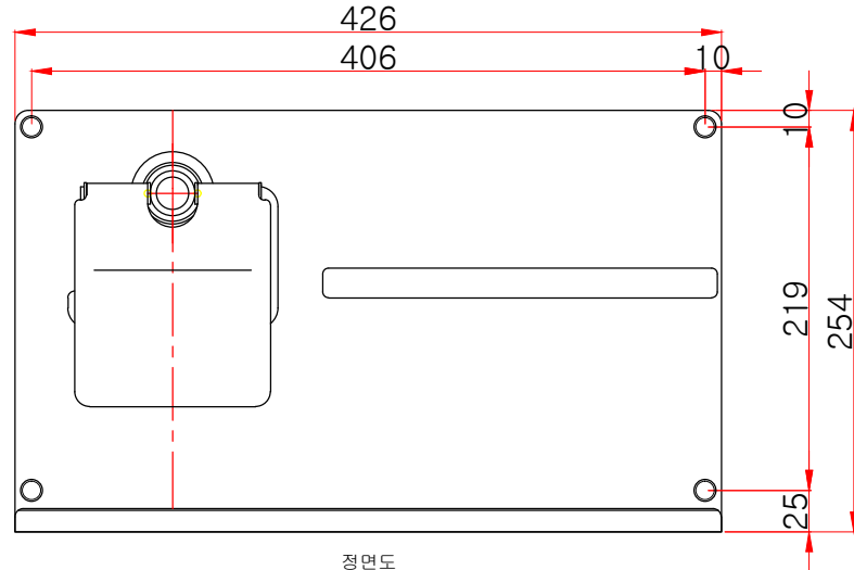
정면도
