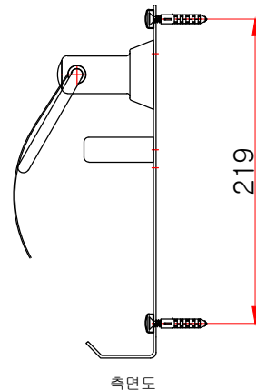
측면도
