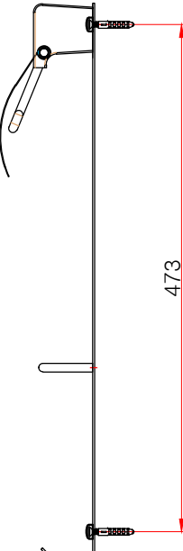
측면도
