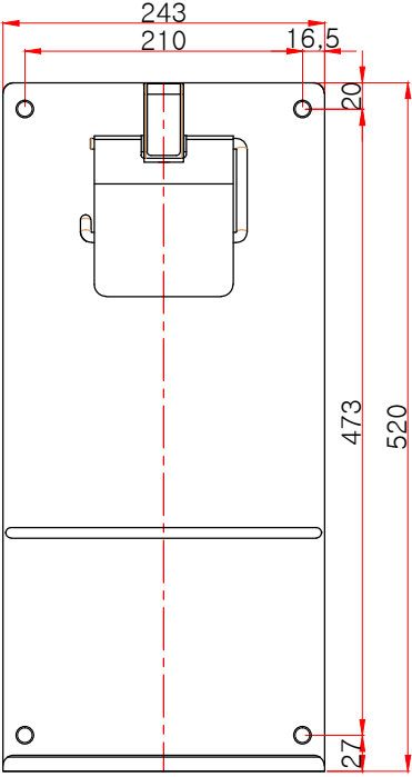
전면도
