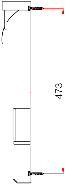
측면도
