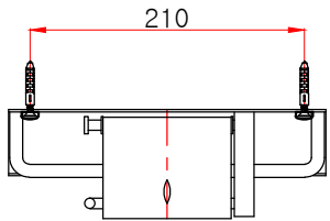
평(상)면도
