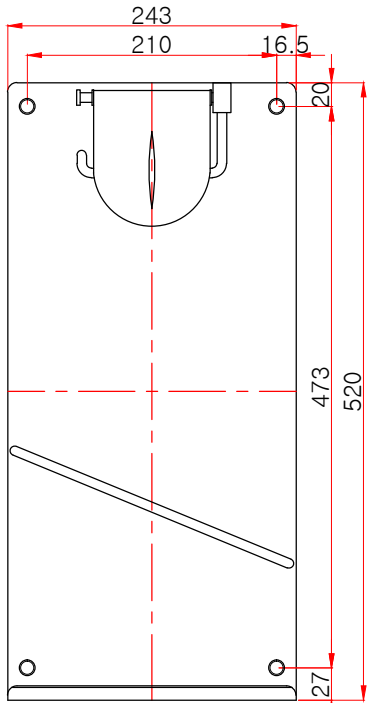
정면도
