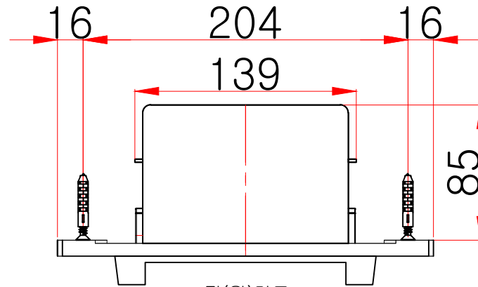
평(윗)면도
