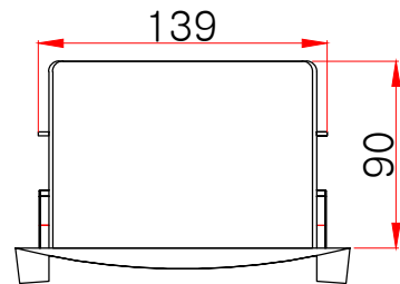
평(윗)면도
