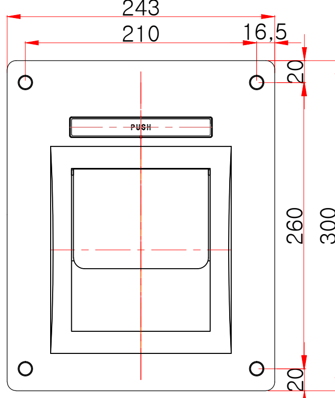
정면도
