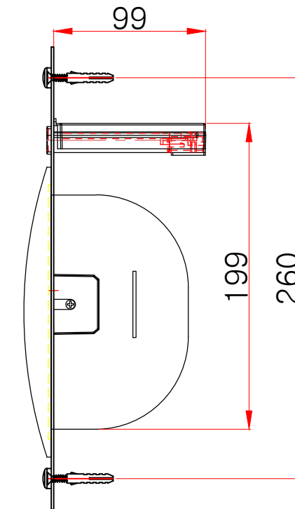
측면도
