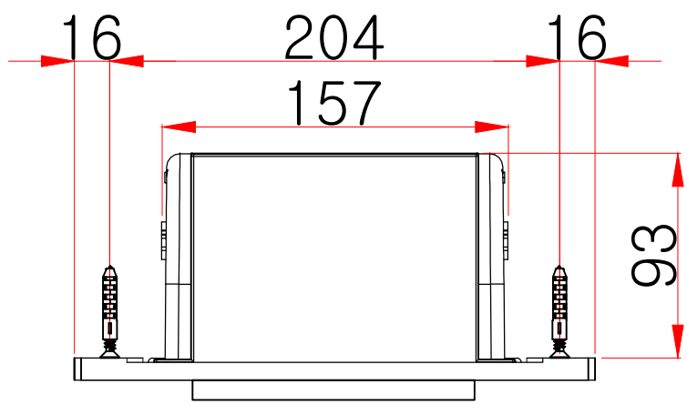
평(윗)면도
