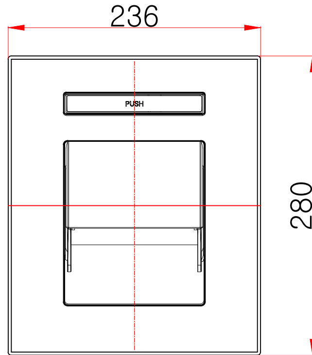
정면도
