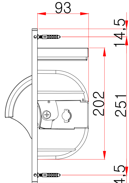
측면도
