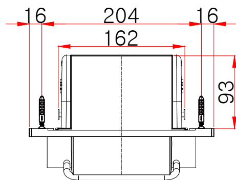
평(위)면도
