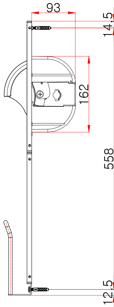
측면도
