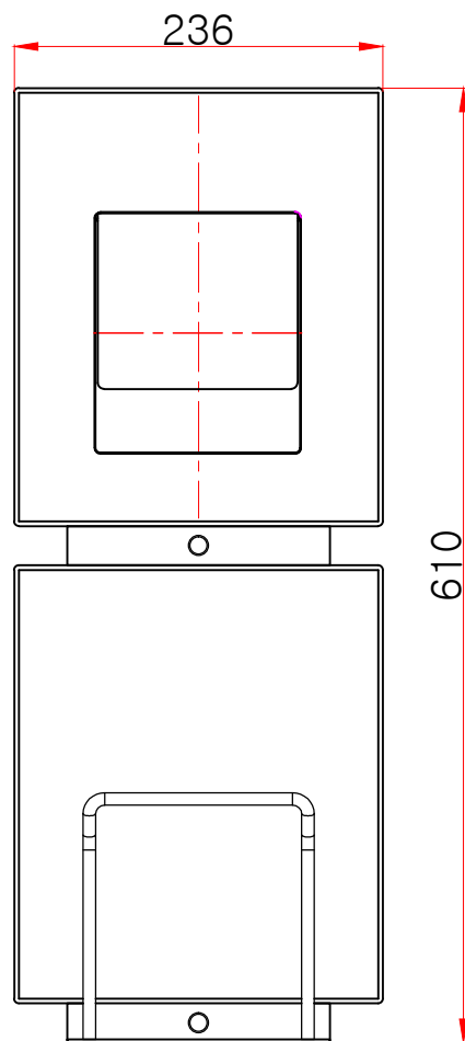
평(윗)면도
