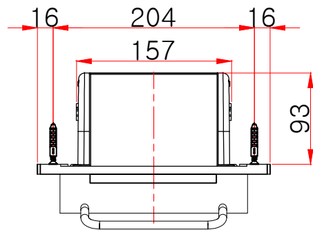
평(윗)면도
