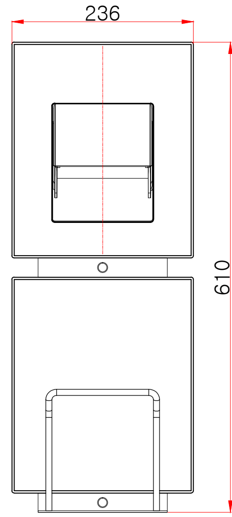
정면도
