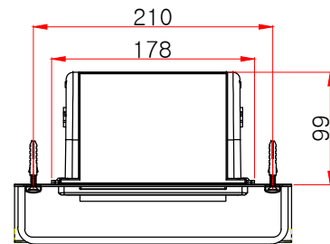
평(위)면도
