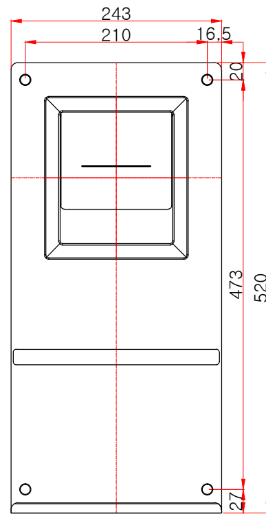
정면도
