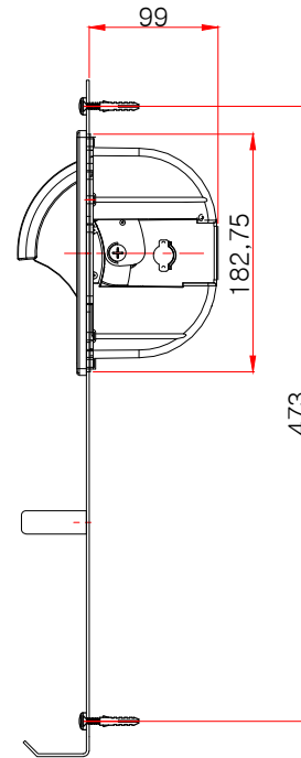
측면도
