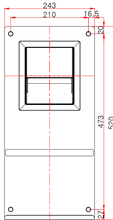
정면도
