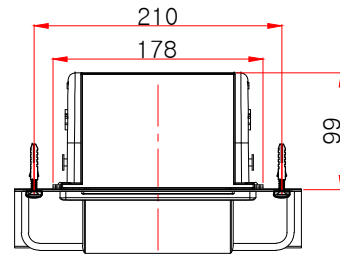
평(위)면도
