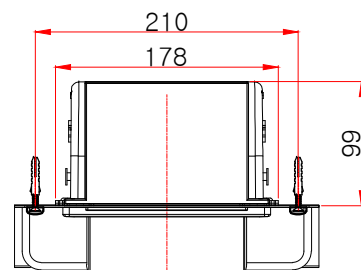
평(위)면도
