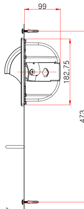
측면도
