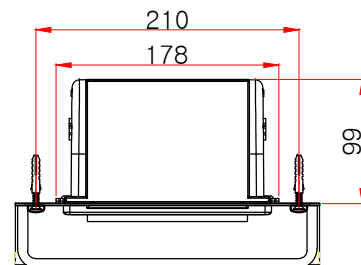
평(위)면도
