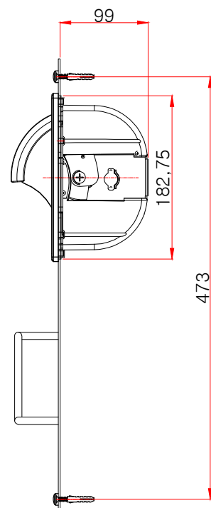
측면도
