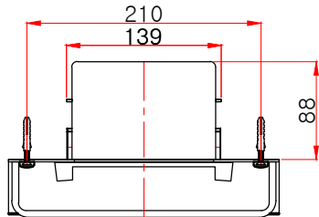
평(위)면도
