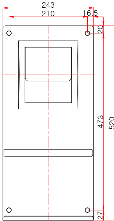
전면도
