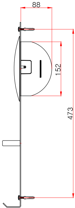
측면도
