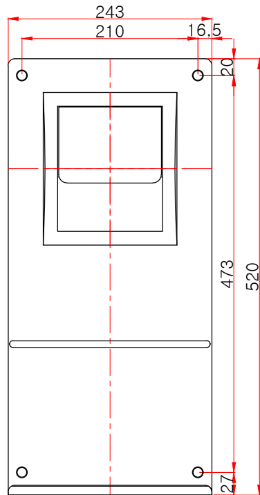
정면도
