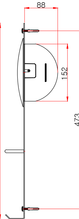
측면도
