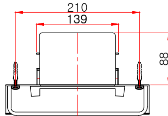
평(윗)면도
