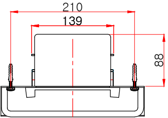
평(상)면도
