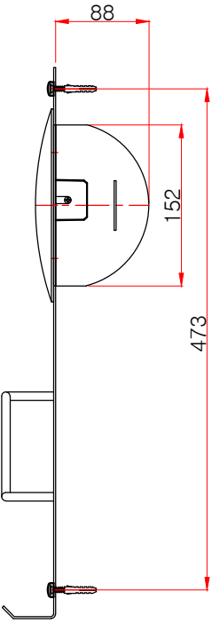
측면도
