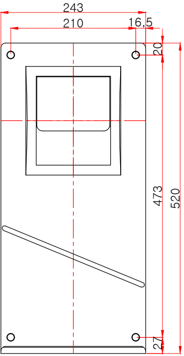
정면도
