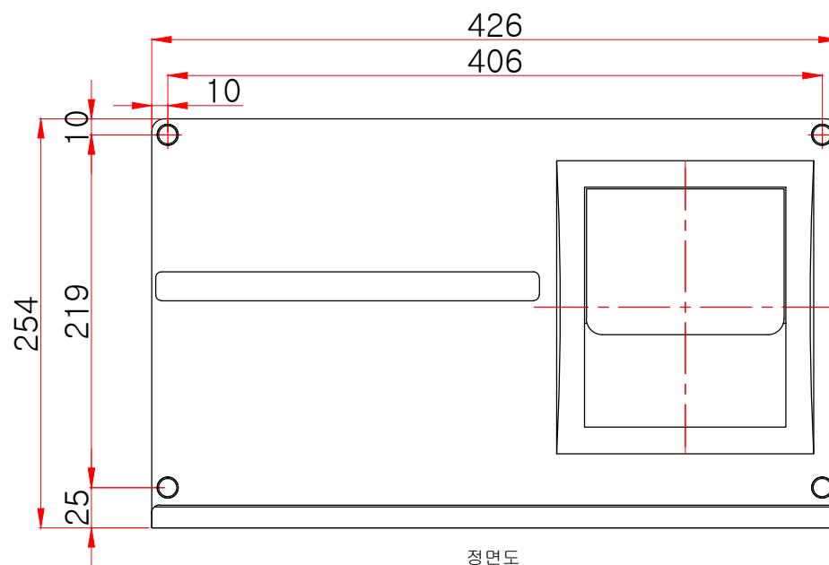
정면도
