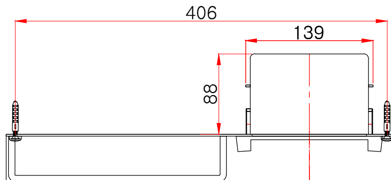
평(윗)면도
