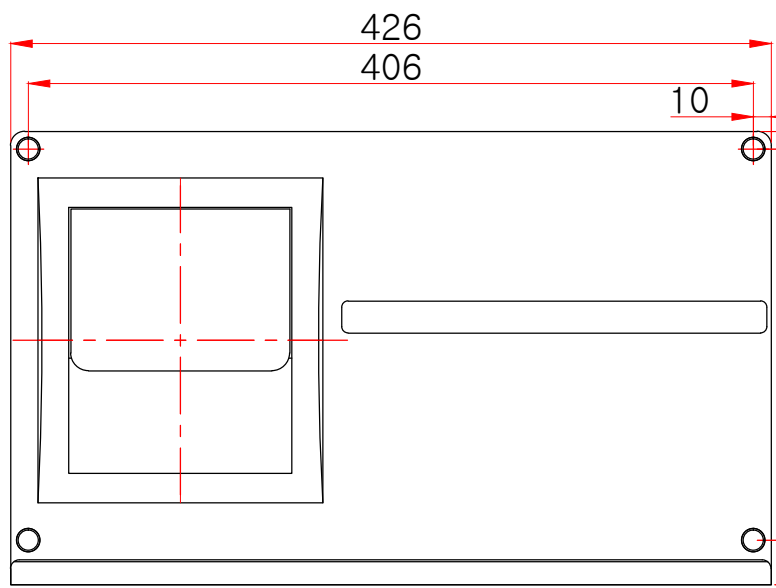
정면도
