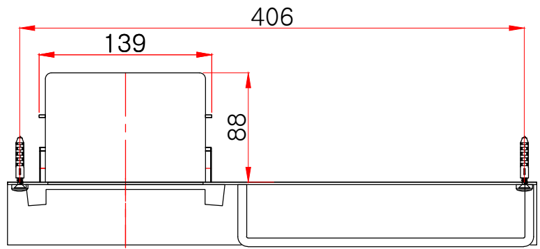
평(윗)면도
