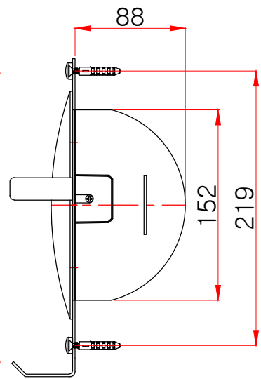
측면도
