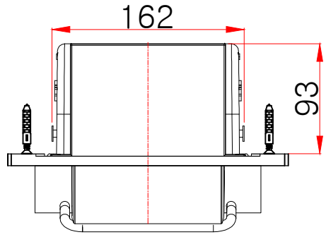
평(위)면도
