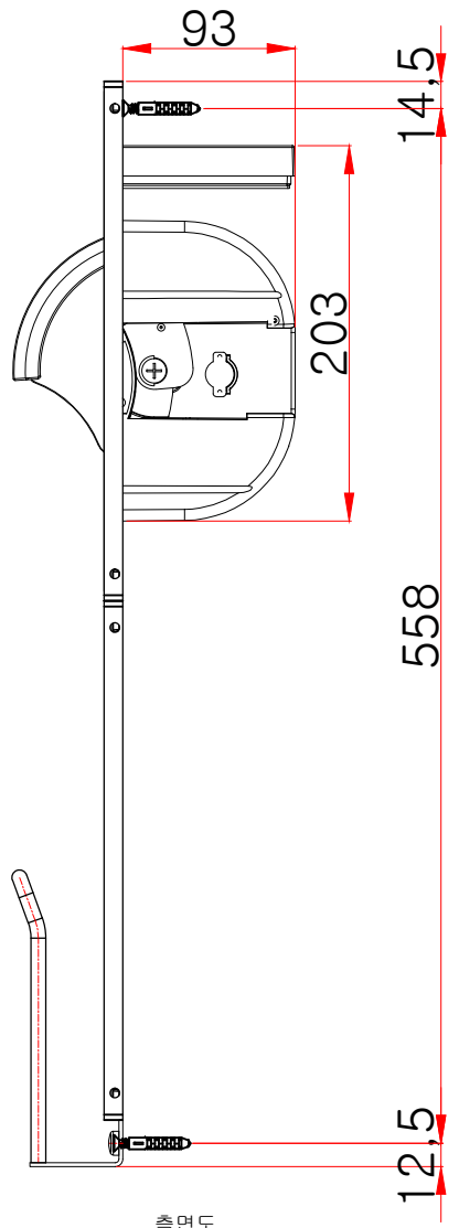
측면도
