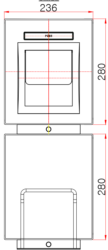
평(위)면도
