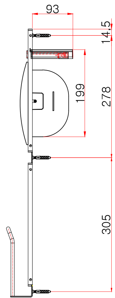
측면도
