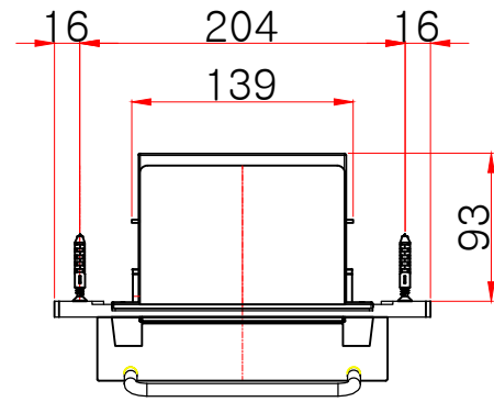
평(위)면도
