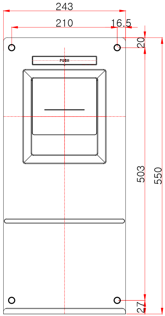
평(상)면도
