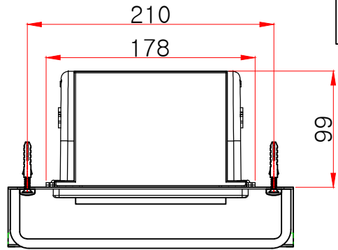
평(상)면도
