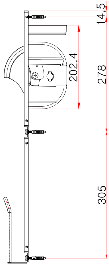
측면도
