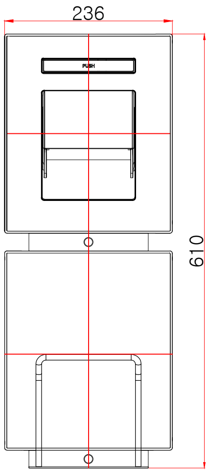
정면도
