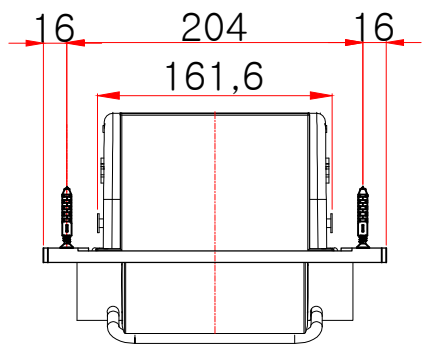
평(윗)면도
