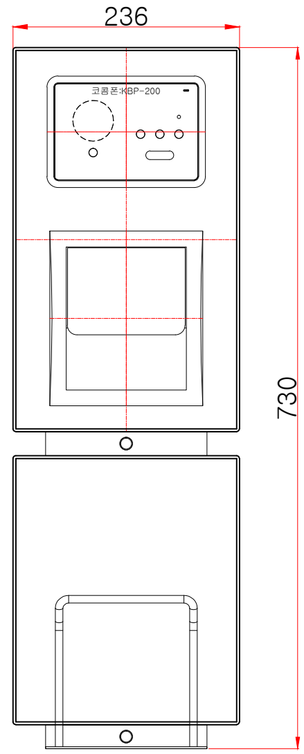
전면도
