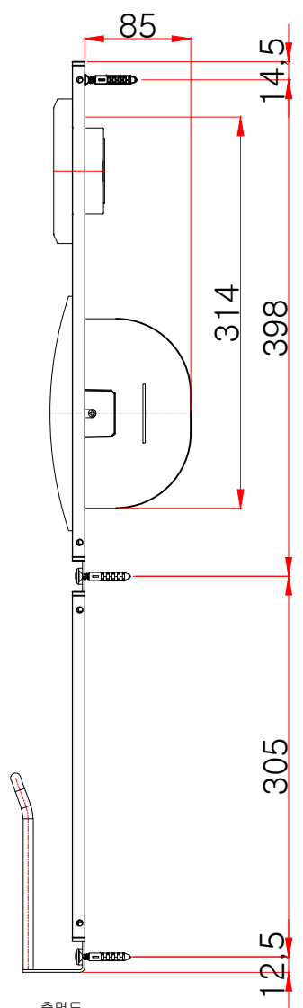
측면도
