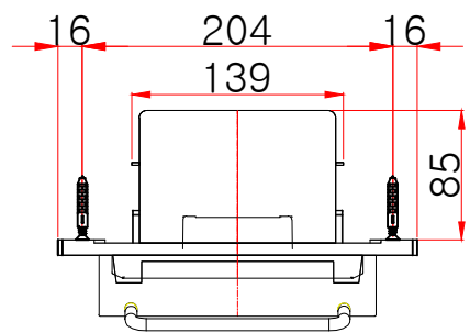
평(위)면도
