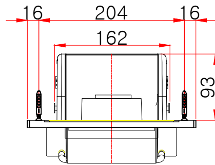
평(위)면도
