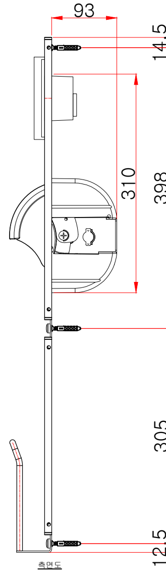
측면도
