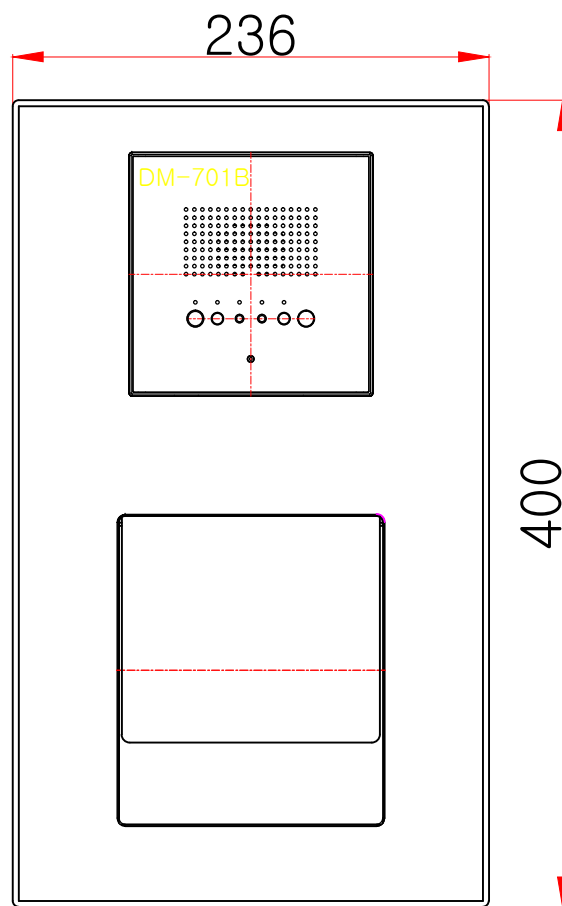
정면도
