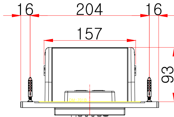
평(윗)면도
