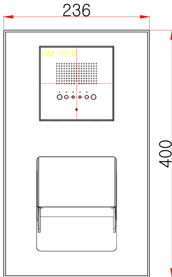
정면도
