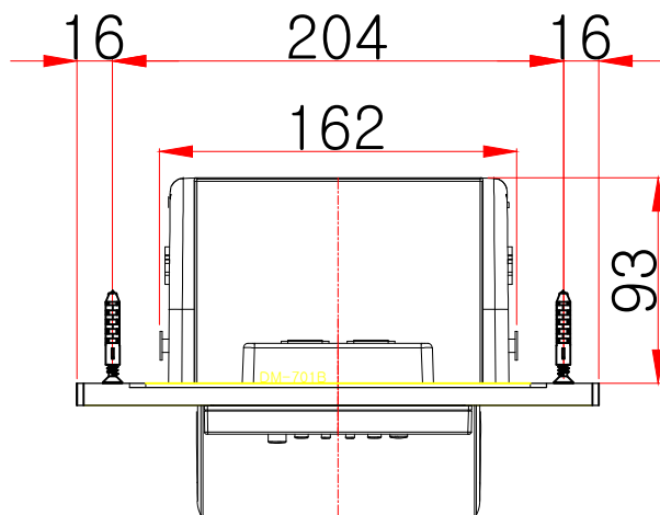
평(윗)면도
