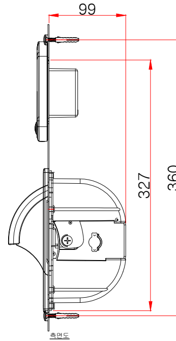
측면도
