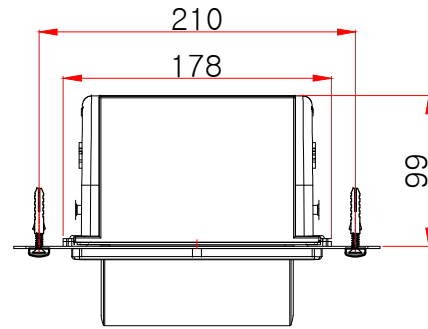
평(위)면도
