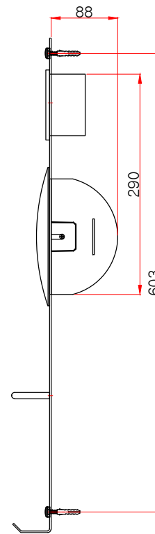
측면도
