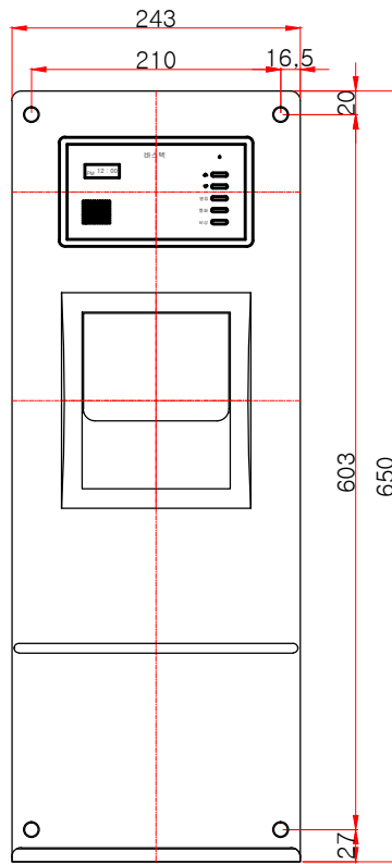
정면도
