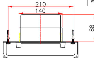
평(상)면도
