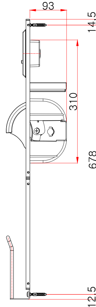
측면도
