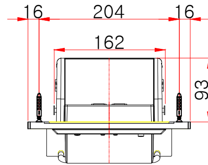
평(위)면도
