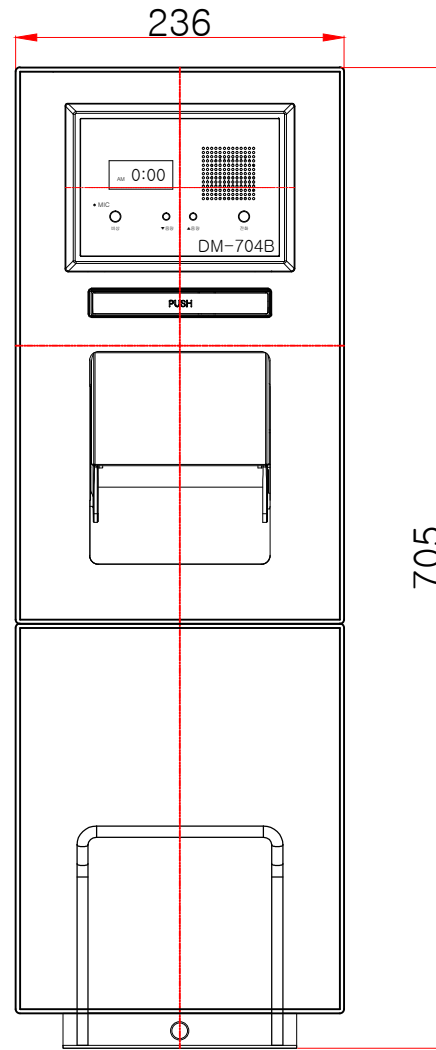
정면도
