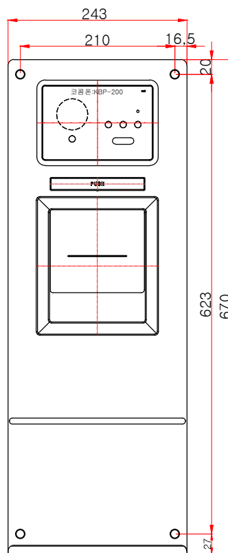
전면도
