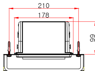
평면도
