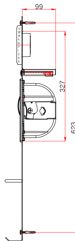
측면도
