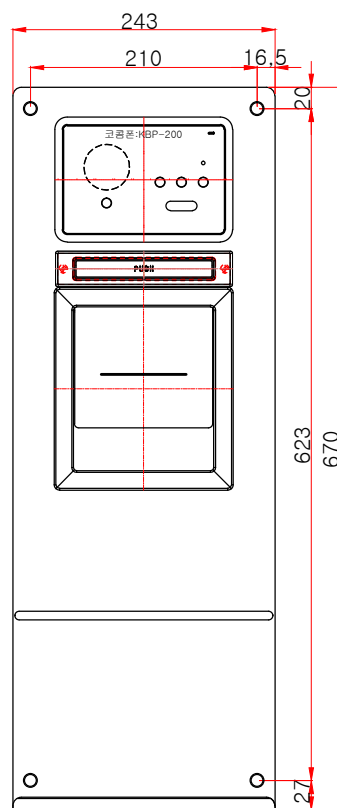
전면도
