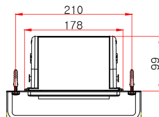
좌(상)면도
