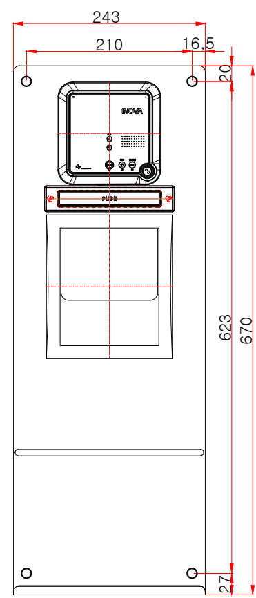
전면도
