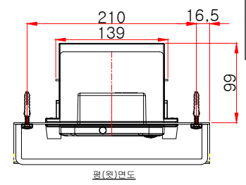
평(상)면도
