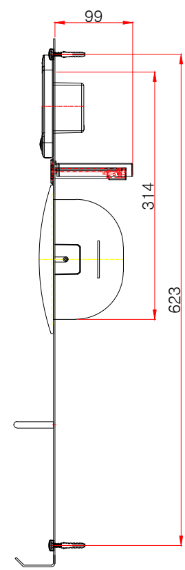
측면도
