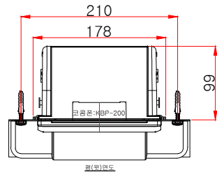
상(하)면도
